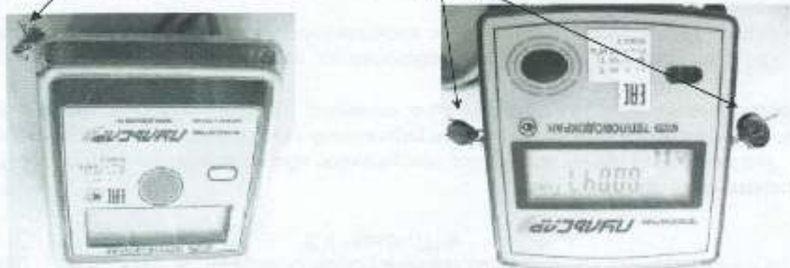
в) схема пломбировки термощетяков с сопротивлением на трубопроводе
